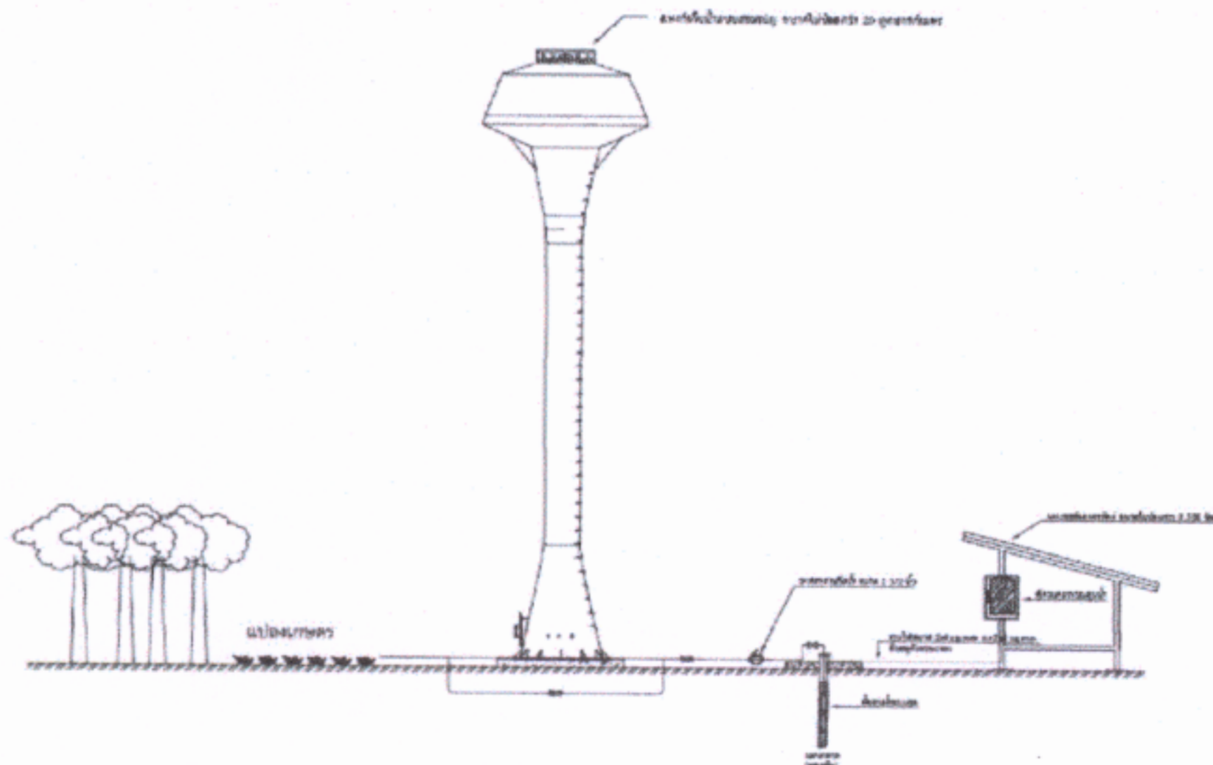
รูปที่ 1. ระบบสูบน้ำด้วยเซลล์แสงอาทิตย์ขนาดไม่น้อยกว่า 2,500 วัตต์ แบบหอดังแชมเปญ สำหรับระบบเกษตร
