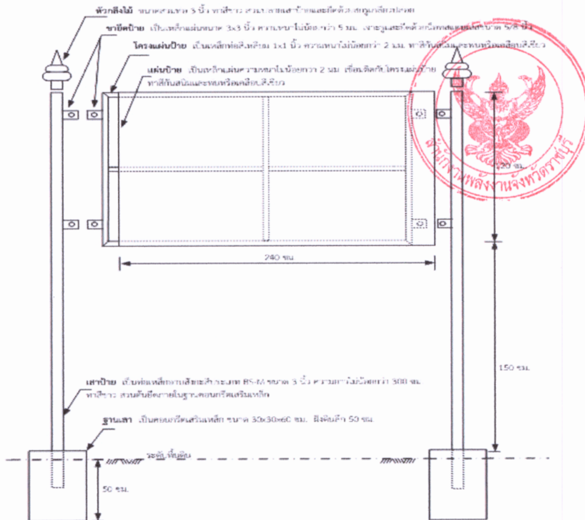
รูปที่ 2 ลักษณะรูปแบบโครงสร้างป้ายชื่อโครงการ (หมายเหตุ รูปไม่ได้แสดงอัตราส่วน)
