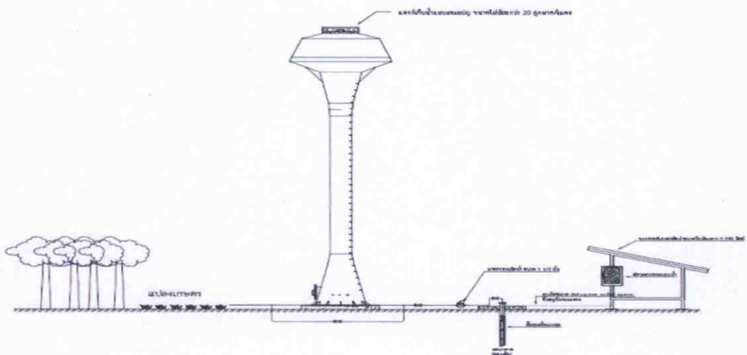
รูปที่ ๑. ระบบสูบน้ำด้วยเซลล์แสงอาทิตย์ขนาดไม่น้อยกว่า ๒,๕๐๐ วัตต์ แบบหอดังแชมเปญ สำหรับระบบเกษตร
